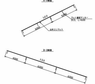
敷設断面図 S=1:100
