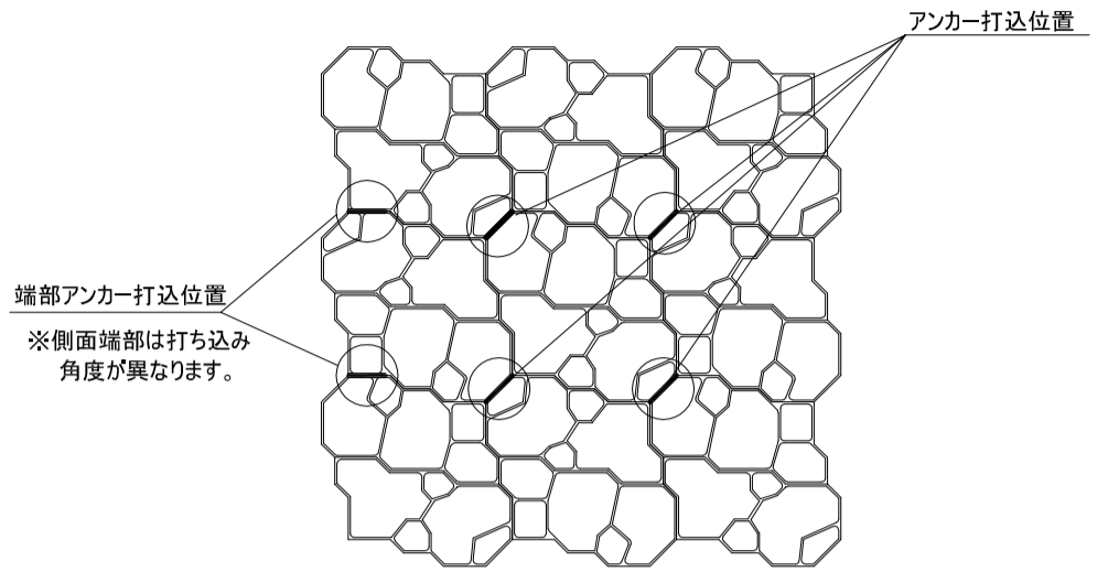
アンカー打込み位置 詳細図
